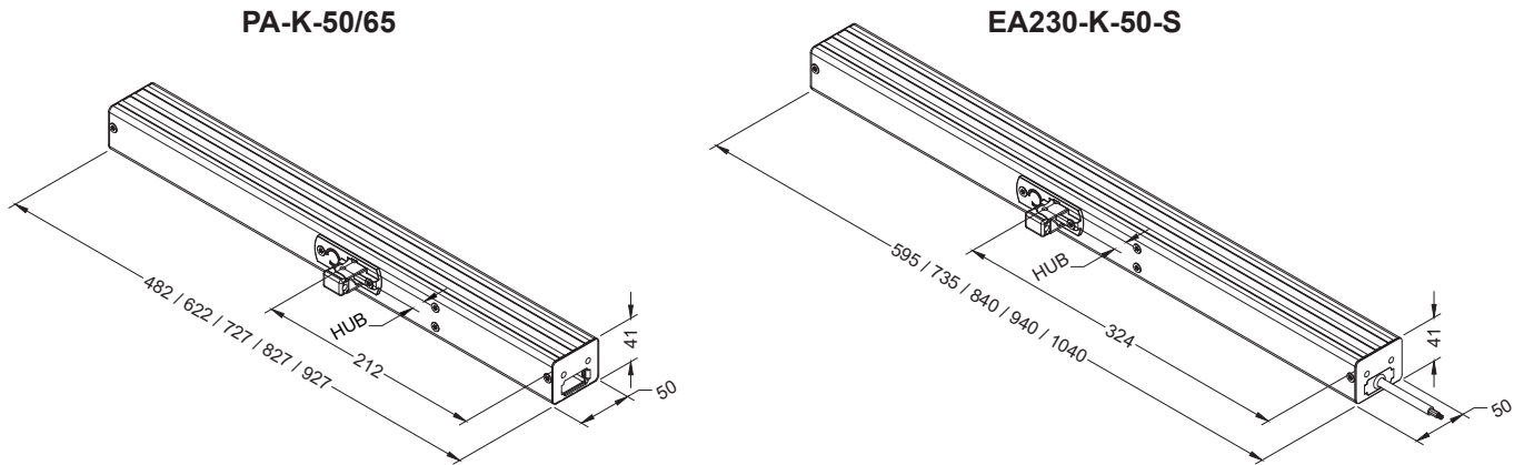
Abbildung 1: Abmessungen Antriebe
