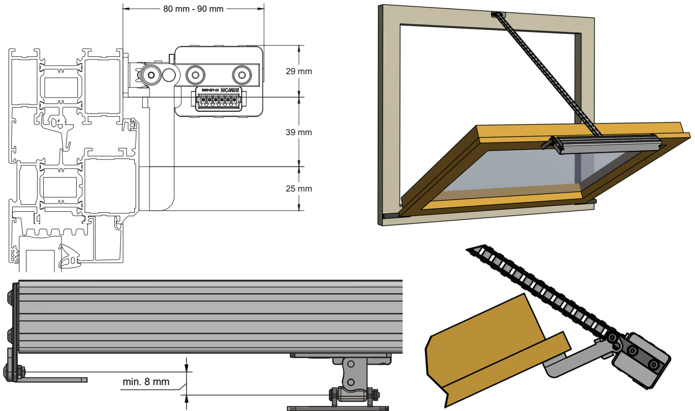
Abbildung 15: Kippflügel
