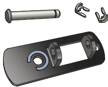
Abbildung 3: Obere Konsole K-K-OK-SK
